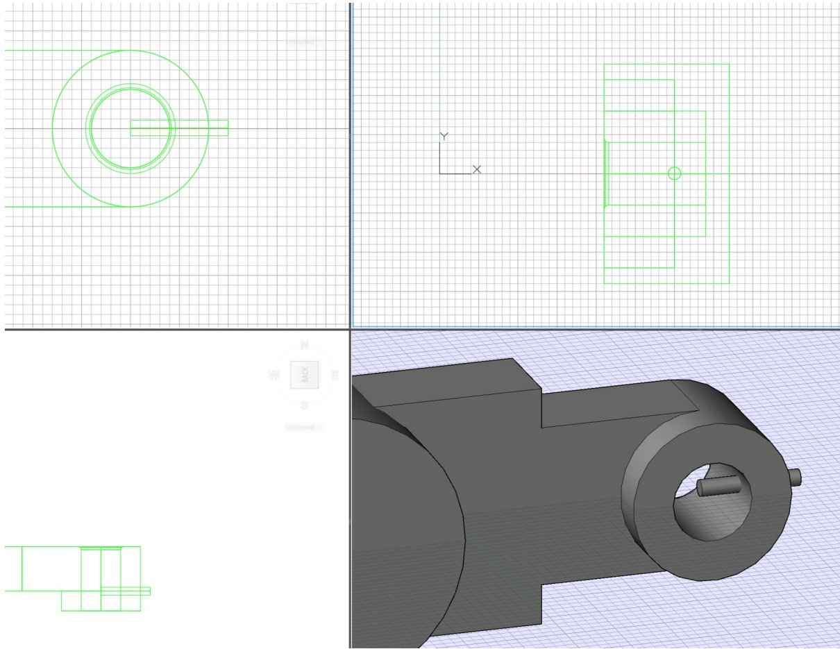
Рисунок 1.7 — Додане коло для віднімання
