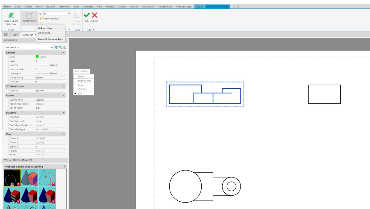
Рисунок 1.10 — Додані види та вимкнені невидимі лінії
