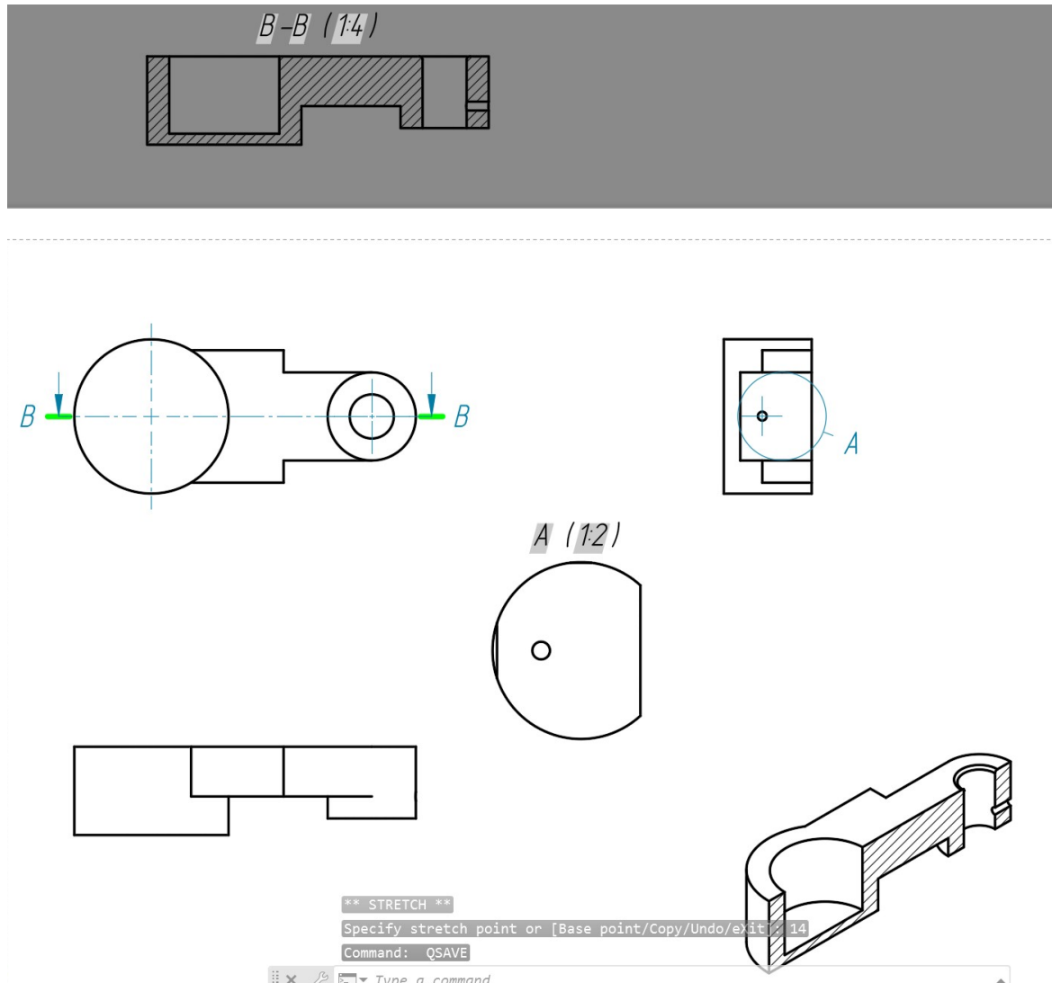
Рисунок 1.11 — Скореговані види і проекція
